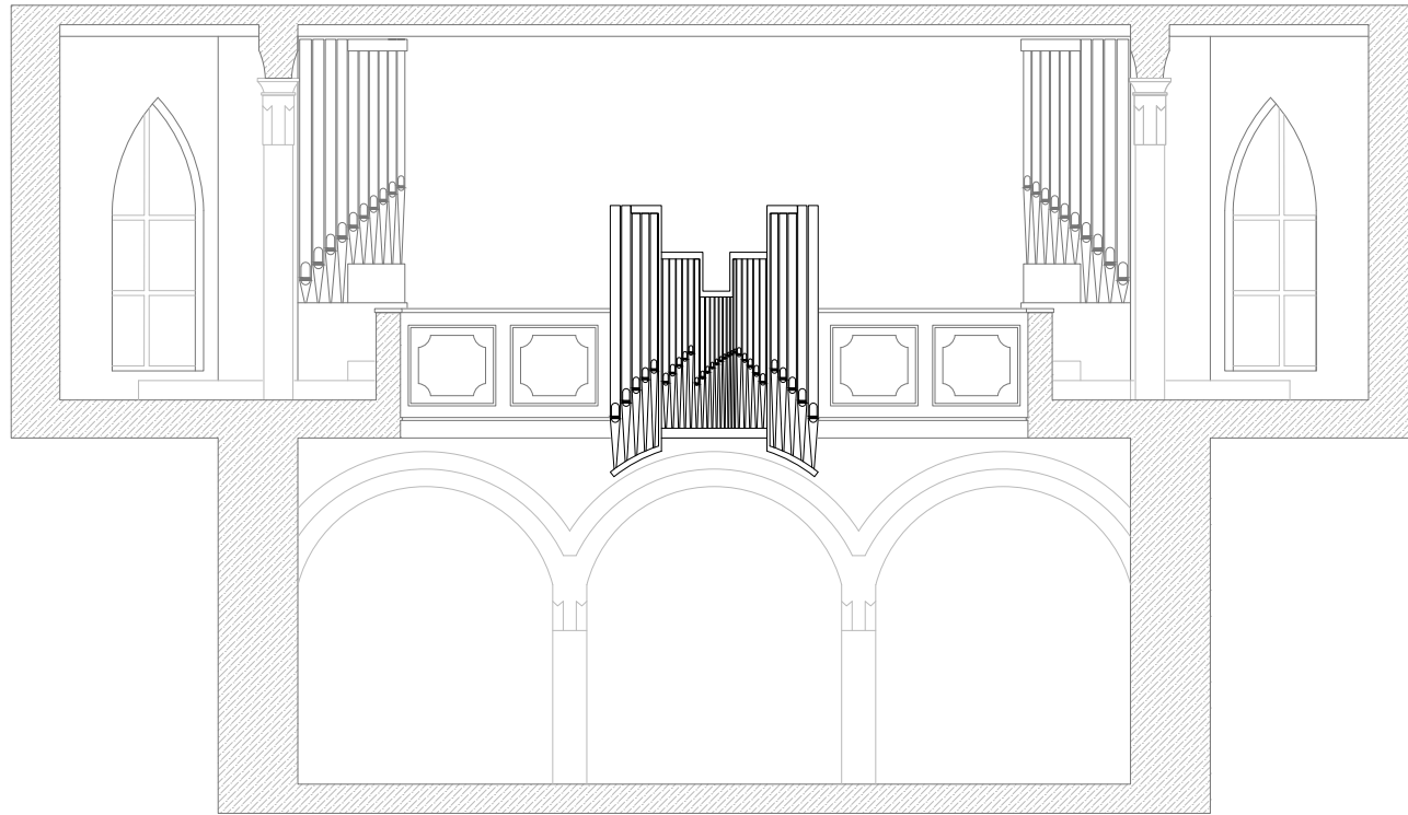
Frontansicht
